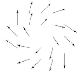
図2 ベクトル場
